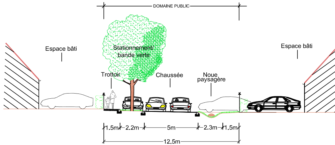
PROFIL BB'
